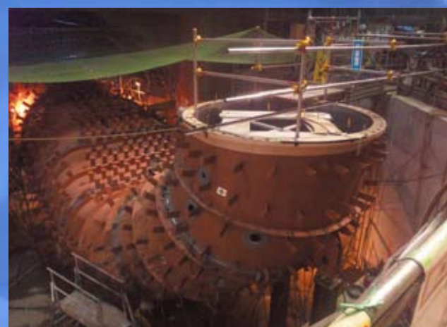
水力発電所 新設工事
