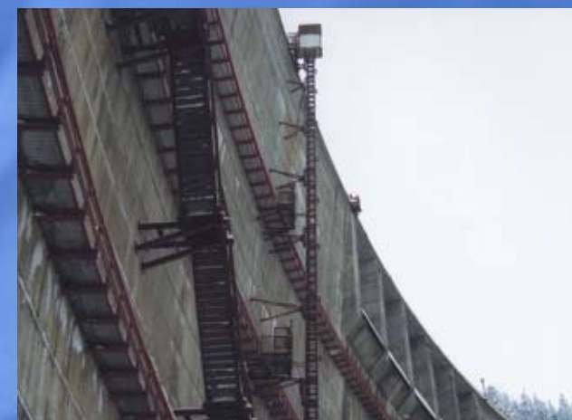
ダム点検用エレベーター交換工事
